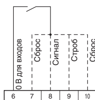
Прим. Вход активизируется при включенном реле
