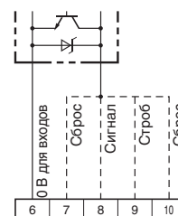
Прим. Вход активизируется при включенном транзисторе
