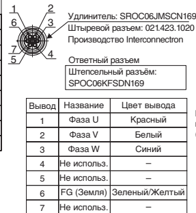
Назначение выводов и параметры разъема линейного серводвигателя
