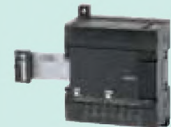
CP1W-MAD42 Входы: 4 (разрешение 12 000) Выходы: 2 (разрешение 12 000)
